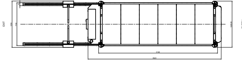
SCHNITTA-A
