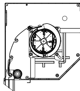
DÉTAIL D ECHELLE 1:5
