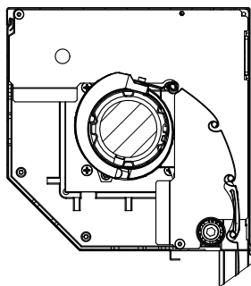
COUPE A-A
