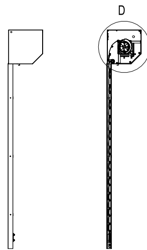
COUPE B-B
